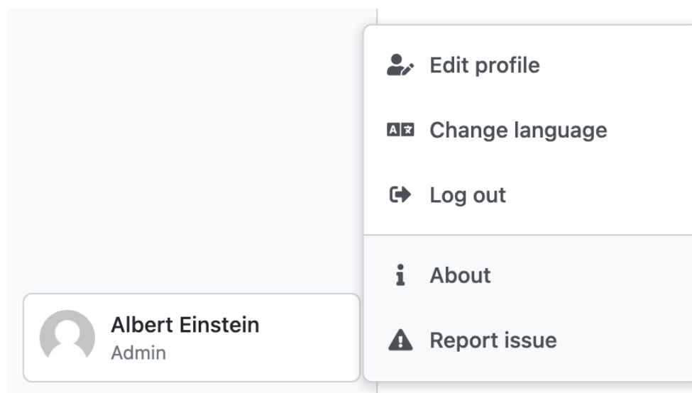
Fig. 76: Profile menu.
